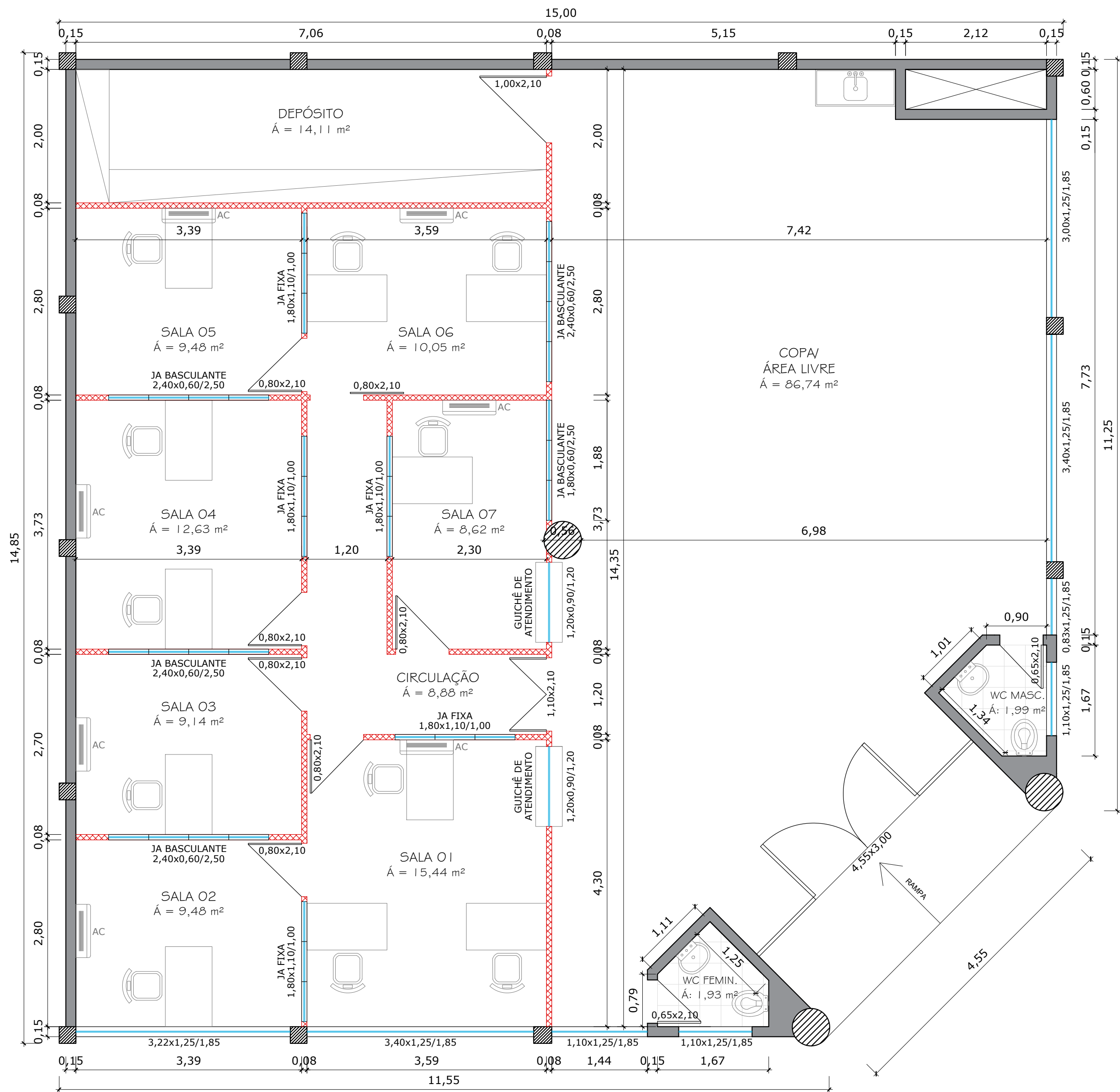
PLANTA DE LAYOUT - PAVILHÃO EXPOSITOR Área Total: 212,54 m² ESCALA 1/50
