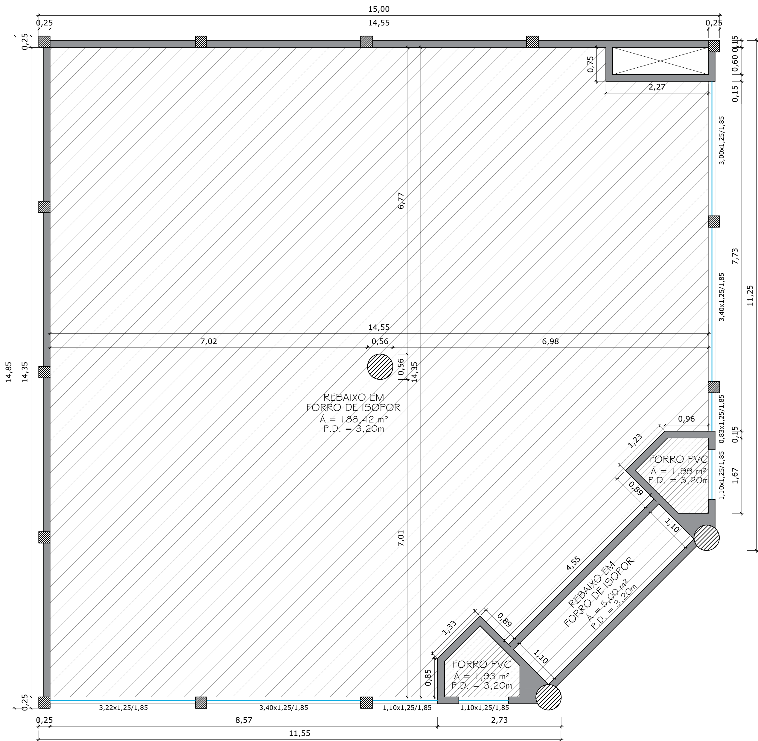
PLANTA DE FORRO - PAVILHÃO EXPOSITOR Área Total: 197,34 m² ESCALA 1/50
