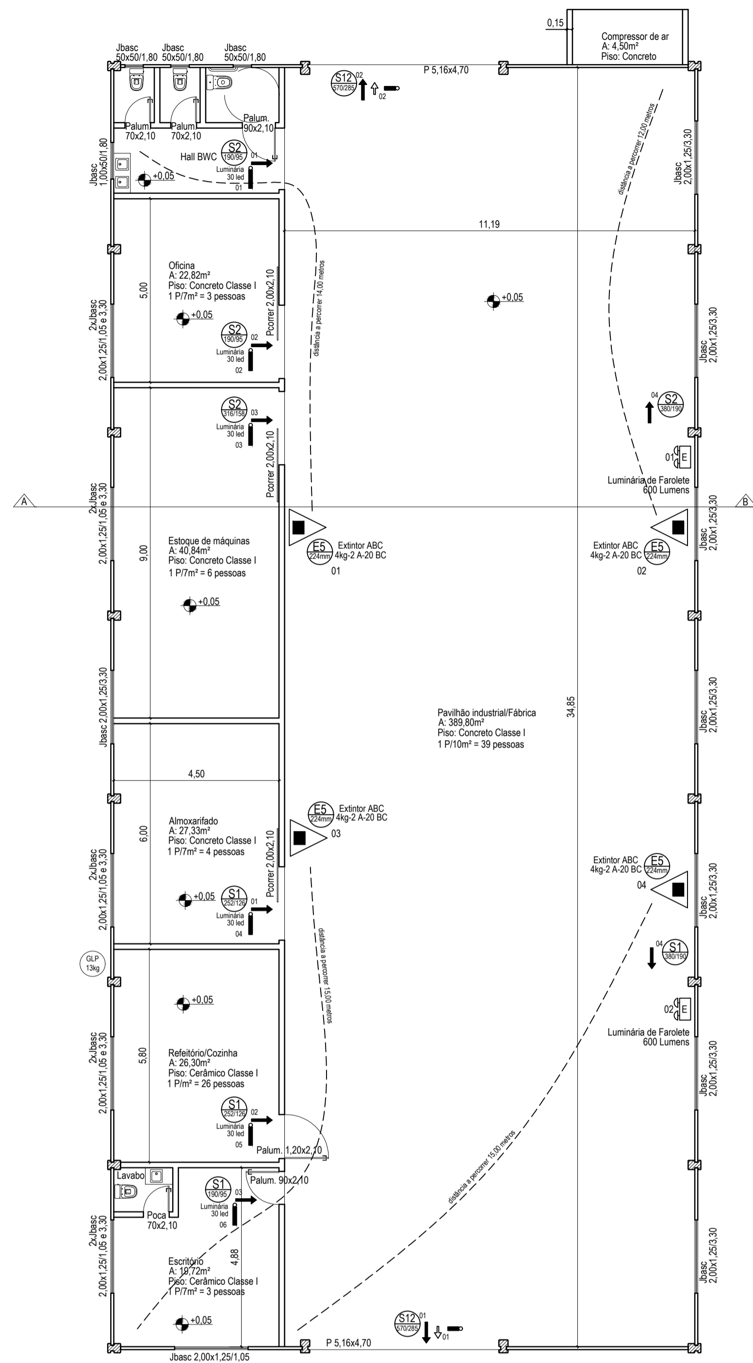
PLANTA BAIXA - PPCI A: 560,12m² Esc.: 1/100
