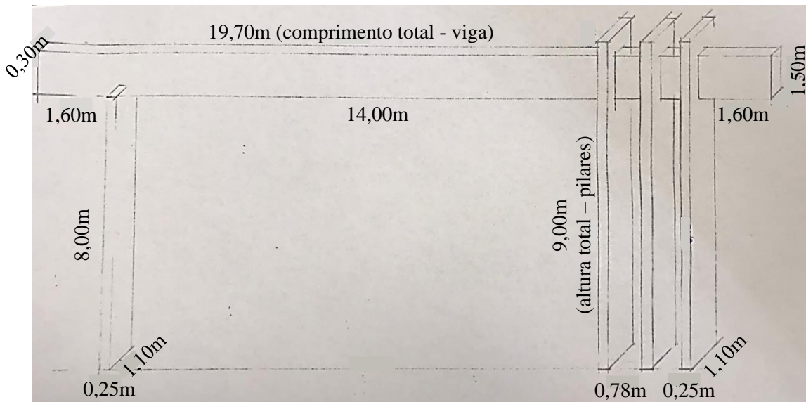
Imagem 03: Esboço com dimensões gerais da estrutura do Pórtico.
